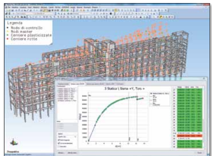
Analisi pushover di una struttura esistente in c.a.
