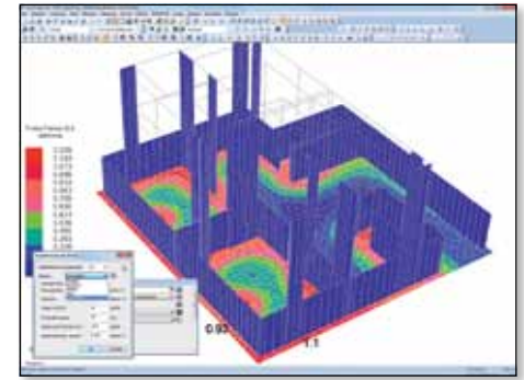
Verifiche geotecniche: calcolo della capacità portante, dello scorrimento e verifica della pressione sul suolo, in figura per una platea.
