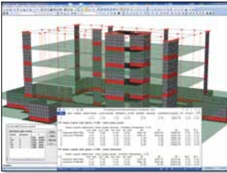
MasterSap esegue il controllo automatico degli effetti del second'ordine per ogni piano e consente, nei casi previsti, di incrementare le forze sismiche.
