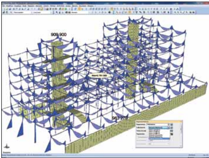
Rappresentazione ed interrogazione dei momenti flettenti in una struttura in c.a., è possibile visualizzare tutte le sollecitazioni e gli stati tensionali derivanti dall'analisi.
