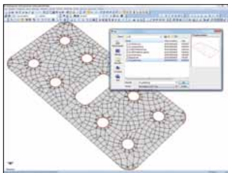
A partire da un disegno caricato e liberamente posizionato nello spazio, con pochi clic si può generare la mesh di una piastra forata.
